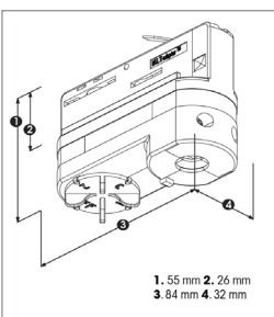
10A Multi-circuit adapter
