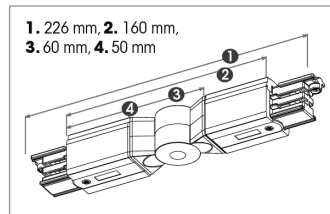
Acessório de união ajustável
