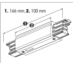
Alimentador eléctrico central
