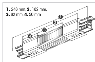
Junta de unión Flexible
