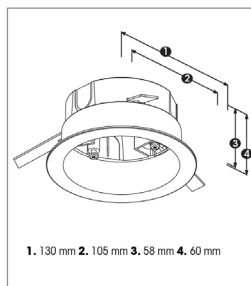
Caja Empotrable para Accesorios de superficie
